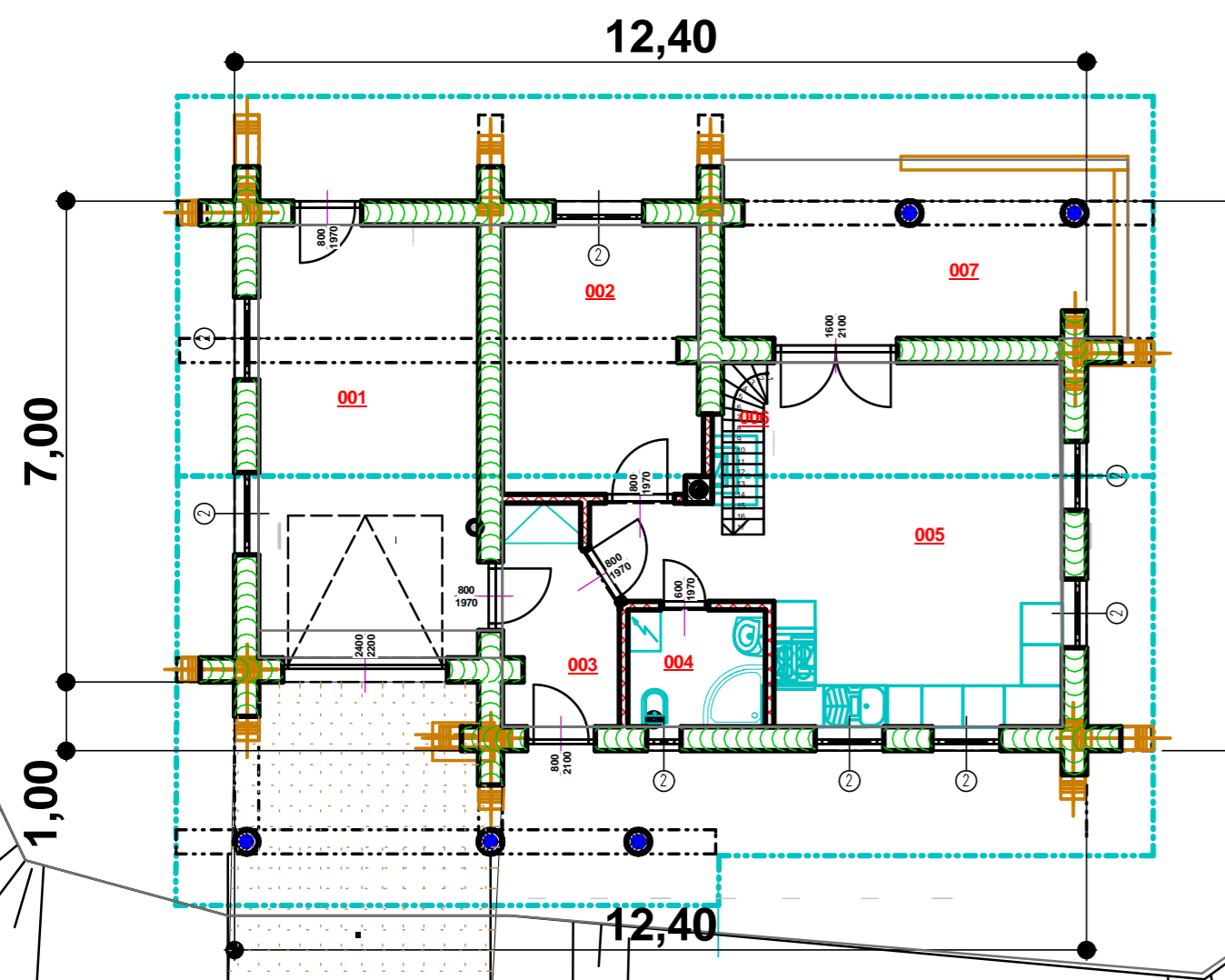
PŮDORYS 1. NP
